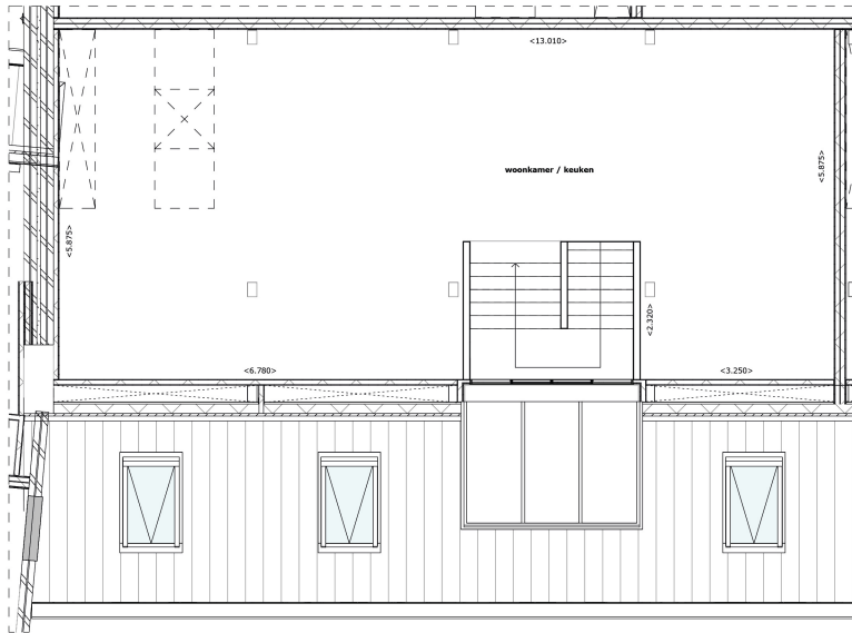
Plattegrond verdieping 04 1:50
